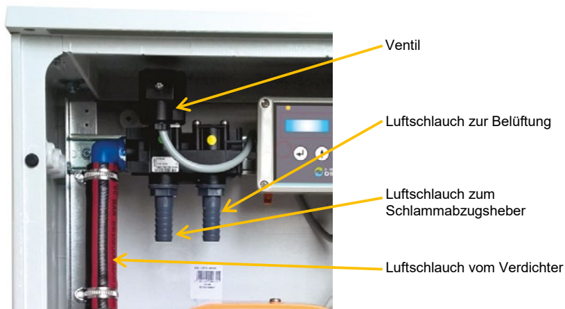
Abbildung 4: Luftanschlüsse
